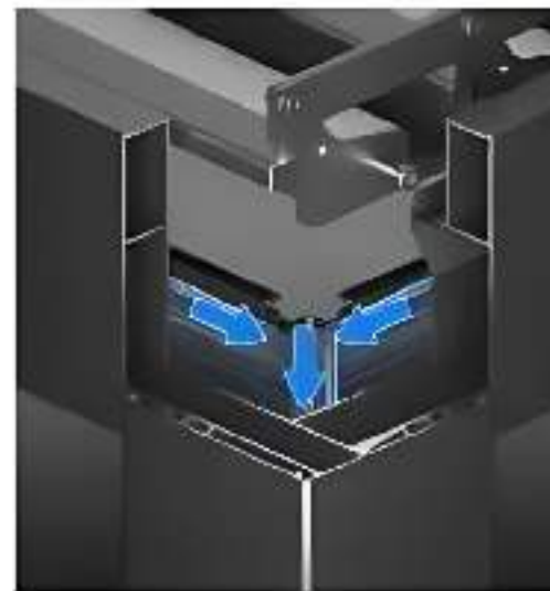
● يتم تدفق المياه إلى العمود
